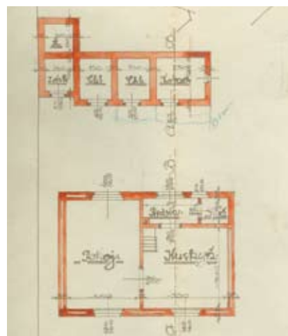
Kopie části stavebního plánu z r. 1925. Takovou vnitřní dispozici měla většina domků čtvrti v Ráji. Stavební plánek zapůjčila paní Anna Fiedlerová
